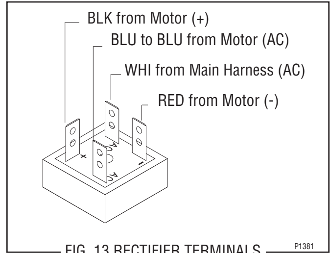
FIG. 13 RECTIFIER TERMINALS
