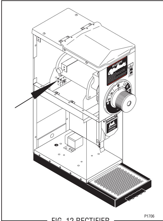
FIG. 12 RECTIFIER
